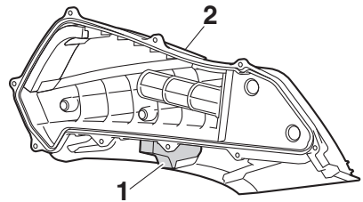
1. Filtro de aire previo 2. Cubierta de la caja del filtro de aire
